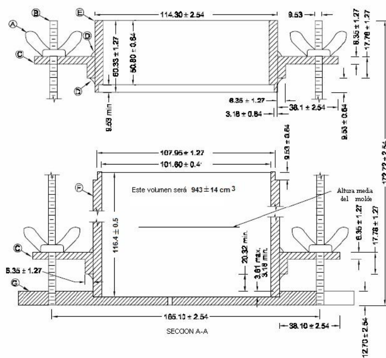
Figura 142 - 1. Molde cilíndrico de 101.6 mm (4.0") para ensayos de suelos
